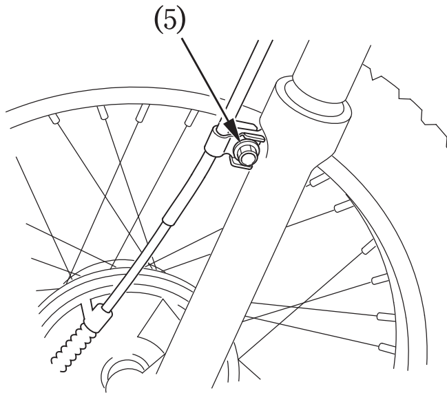
(5) Cable guide bolt
